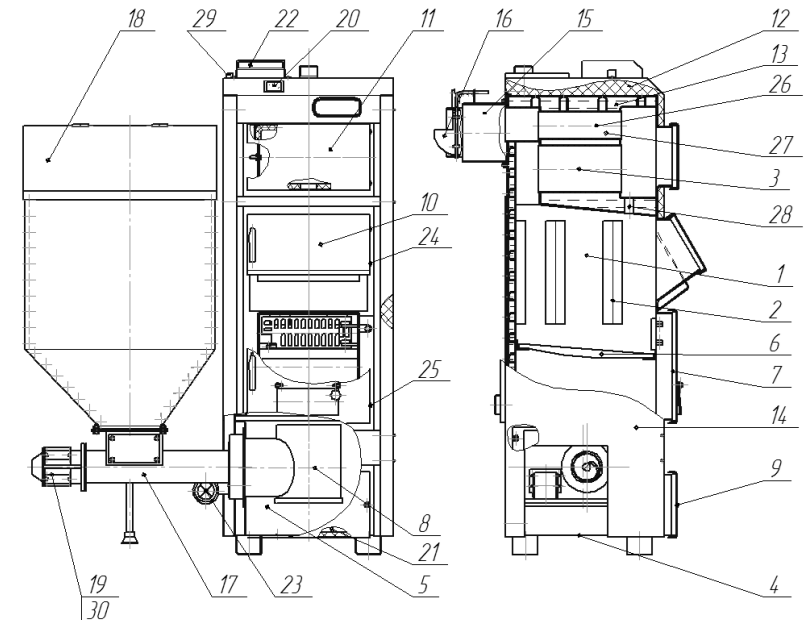
Рис. 1. Апарат опалювальний твердопаливний водогрійний АОТВ 20А.
